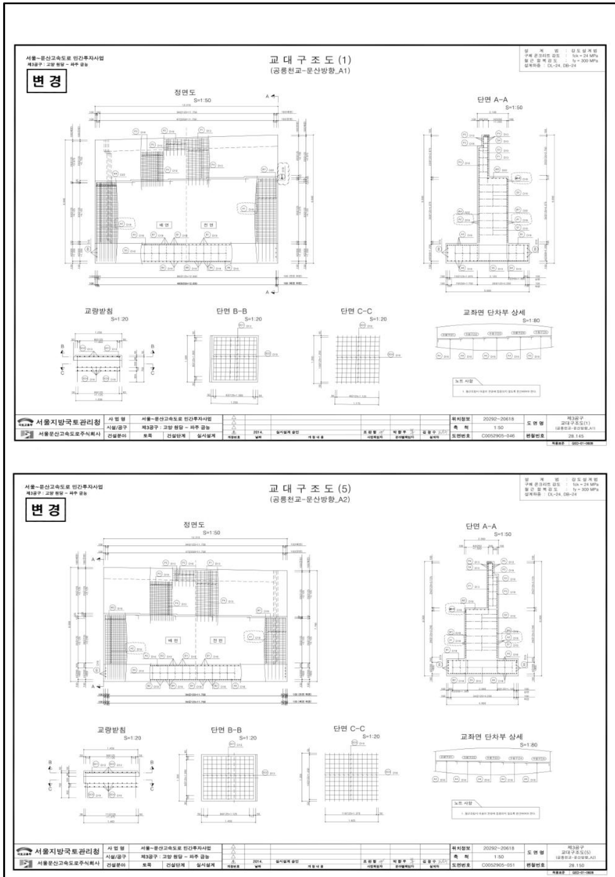
【그림 35.1.9】 교대 배근도
