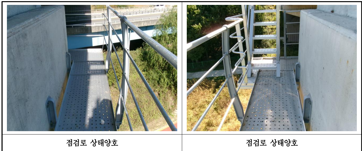
【사진 35.3.26】 교량 점검시설 손상현황
