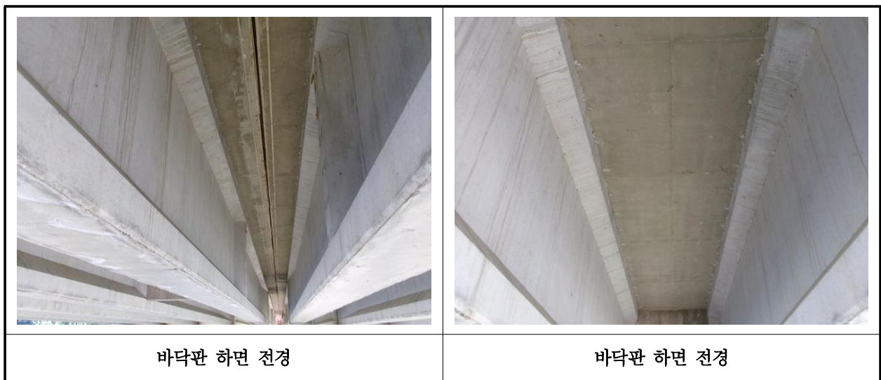
【사진 35.3.2】 바닥판하면 전경
