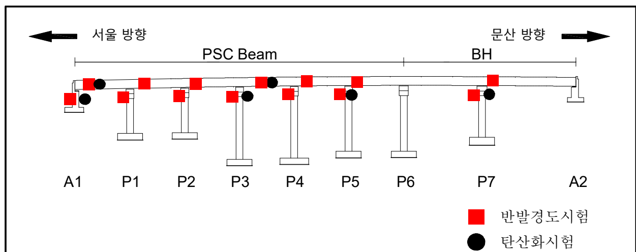
【그림 35.4.1】 콘크리트 내구성조사 위치도
